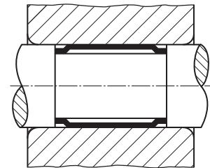
Zentrierter Einbau, Form R0820
