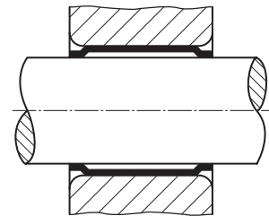
Freier Einbau, Form R0820
