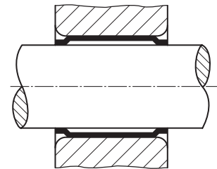
Freier Einbau, Form R0820 System Einheitsbohrung
